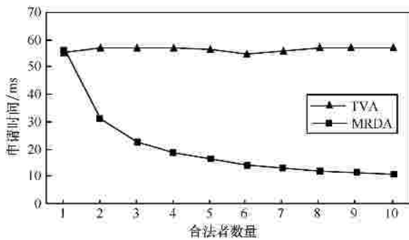
图 13 MRDA 与 TVA 的平均权证请求时间对比
